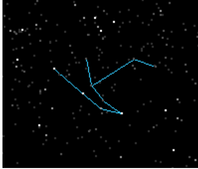
Resim 13-3: Andromeda takımyıldızının gökyüzündeki görüntüsü
