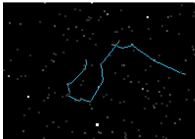
Resim 11-2: Aquarius takımyıldızının gökyüzündeki görüntüsü
