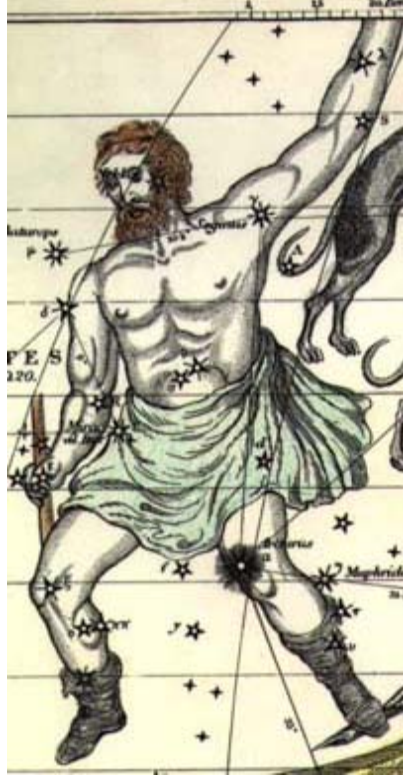
Resim 6-2: Boötes takım yıldızının temsili resmi.
